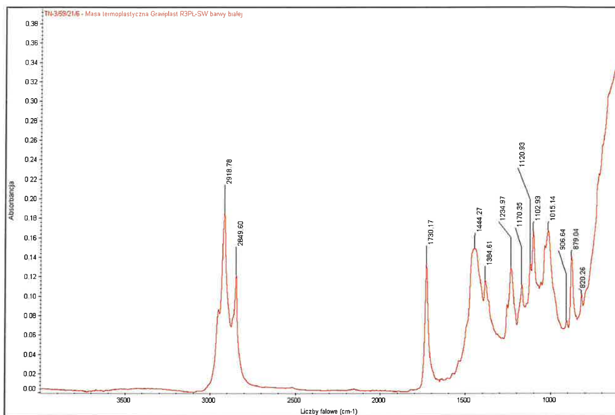
Rysunek 2 - Widmo w podczerwieni masy termoplastycznej GRAVIPLAST 30 barwy białej.
